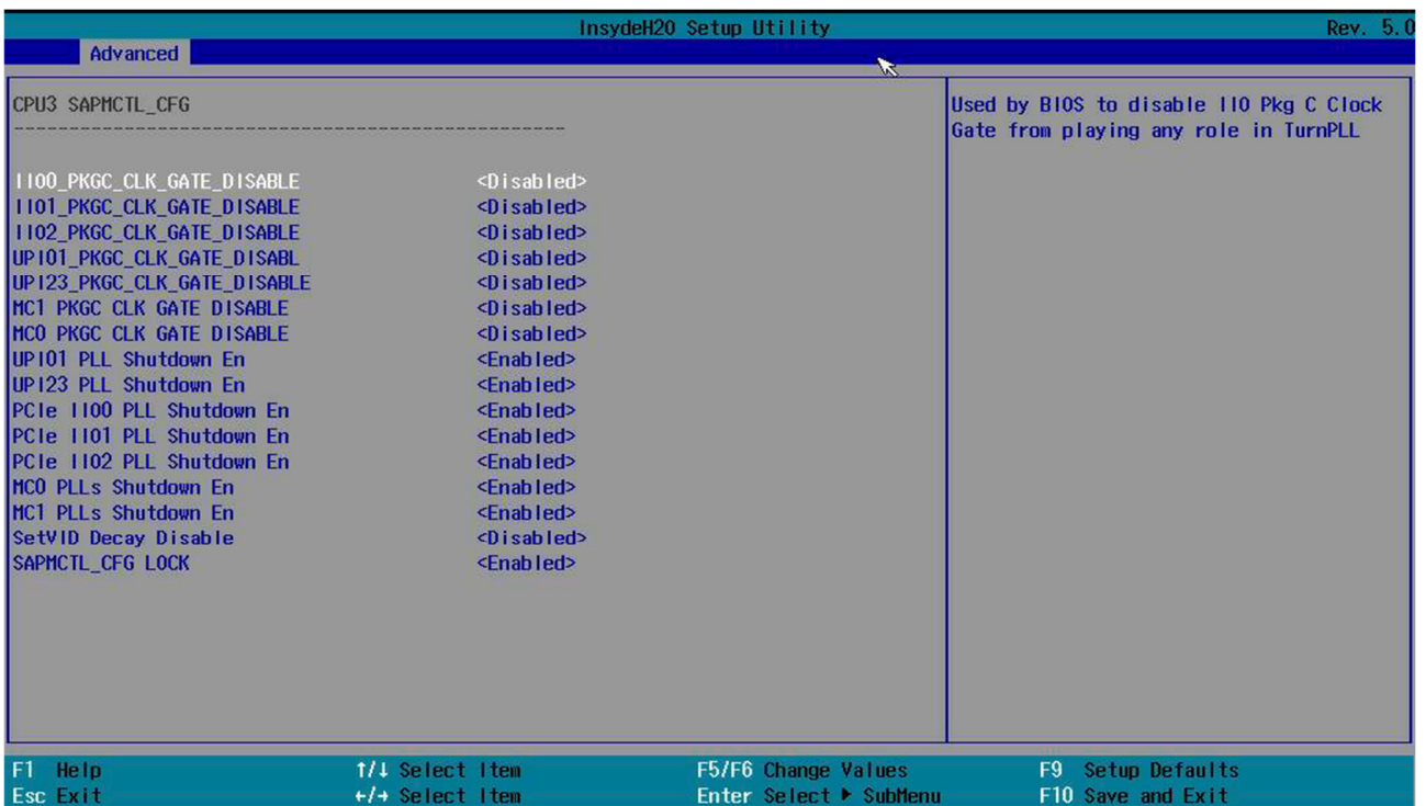
Рисунок 2.42. «CPU3 SAPMCTL_CFG»
