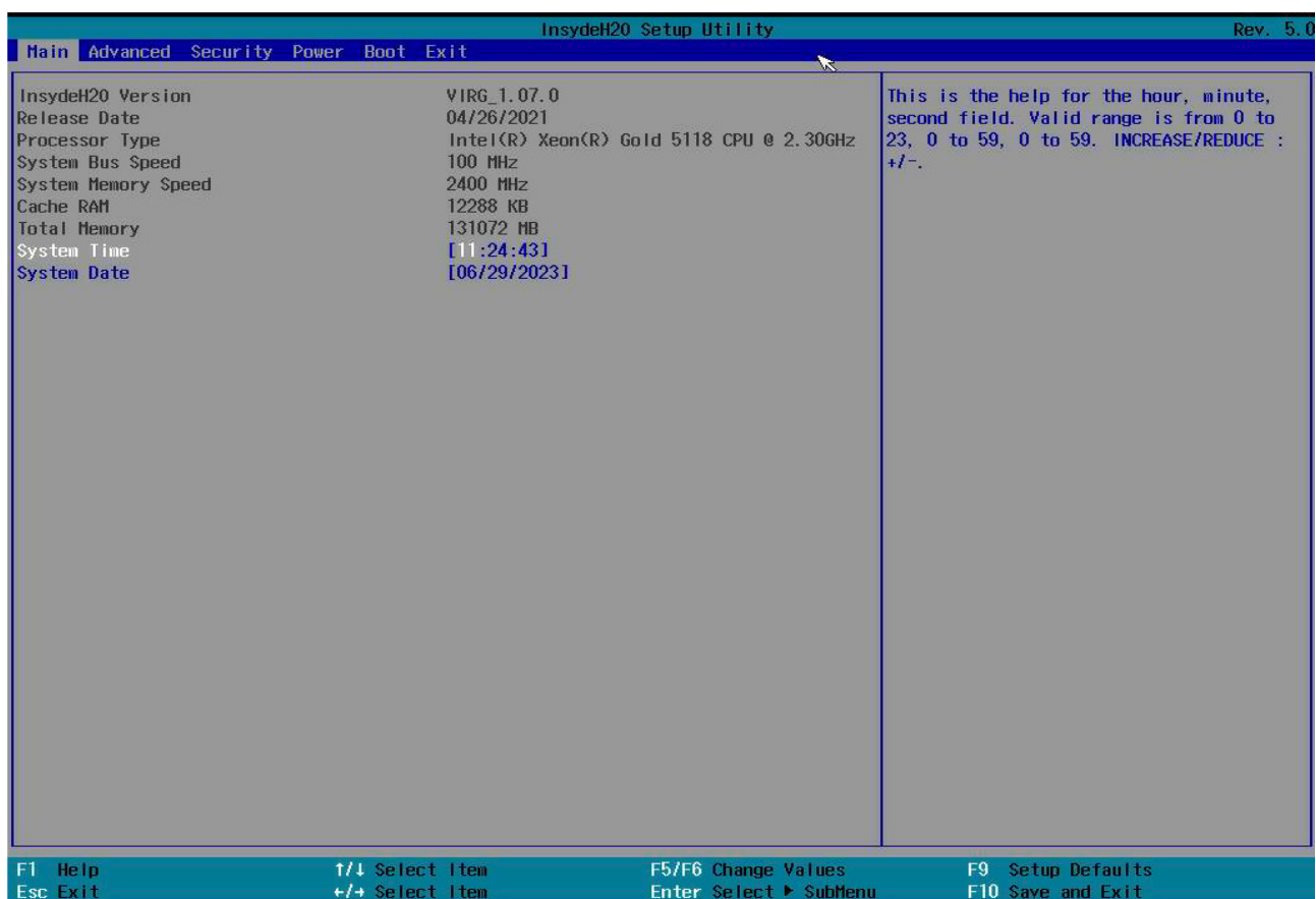
Рисунок 2.1. Вкладка «Main»
