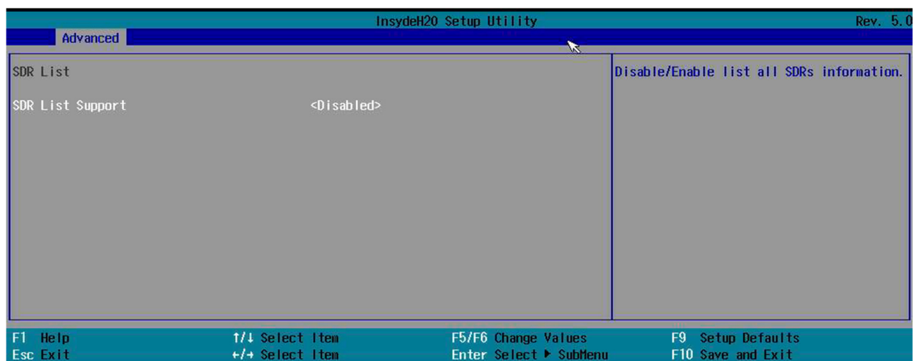
Рисунок 2.57. «SDR List»
