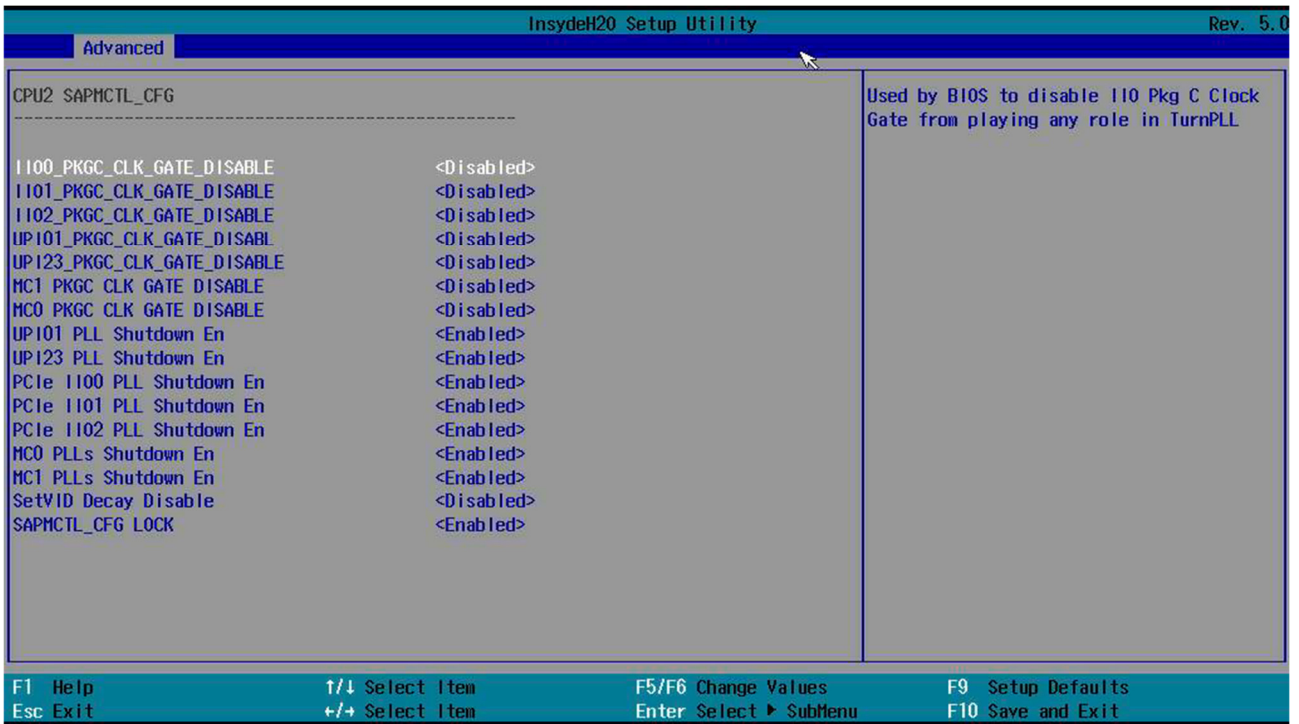
Рисунок 2.41. «CPU2 SAPMCTL_CFG»
