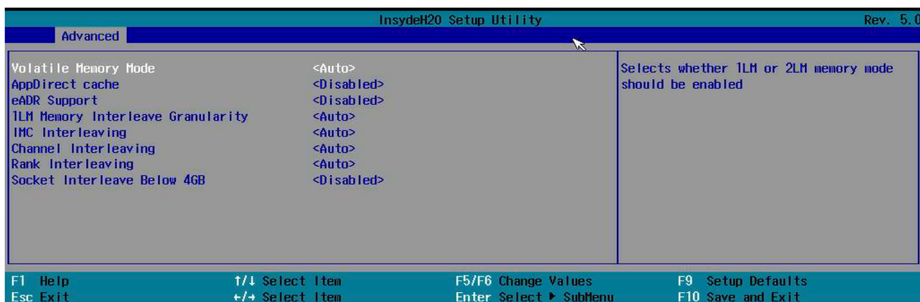
Рисунок 2.15. «Memory Map»
