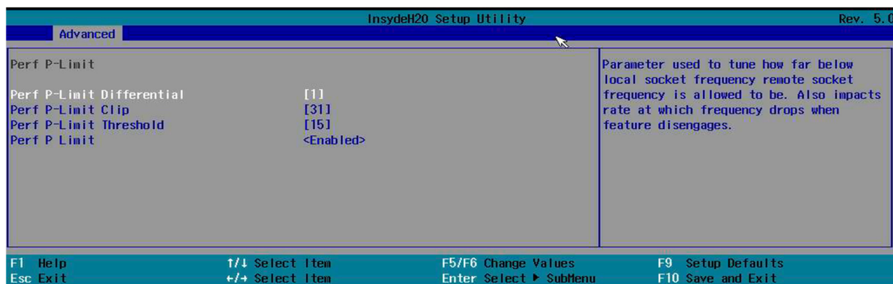
Рисунок 2.34. «Perf P-Limit»
