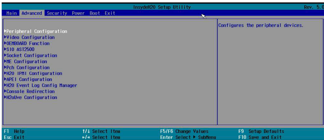
Рисунок 2.2. Вкладка «Advanced»
