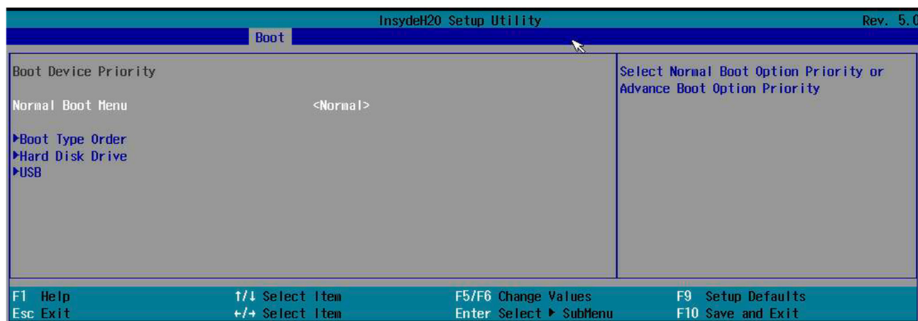
Рисунок 2.72. «Legacy»
