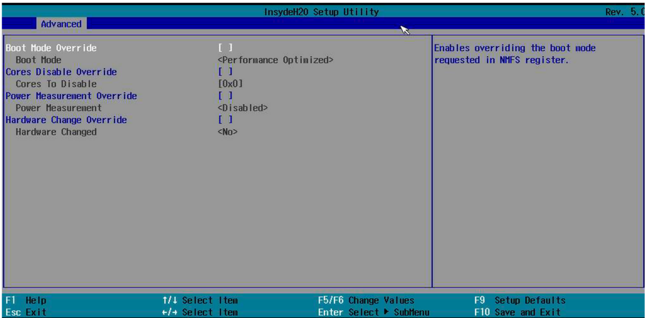
Рисунок 2.48. «NM Configuration»
