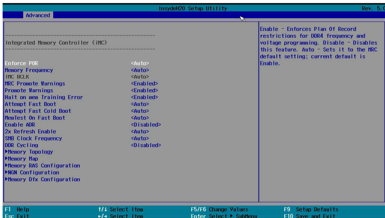
Рисунок 2.13. «Memory Configuration»
