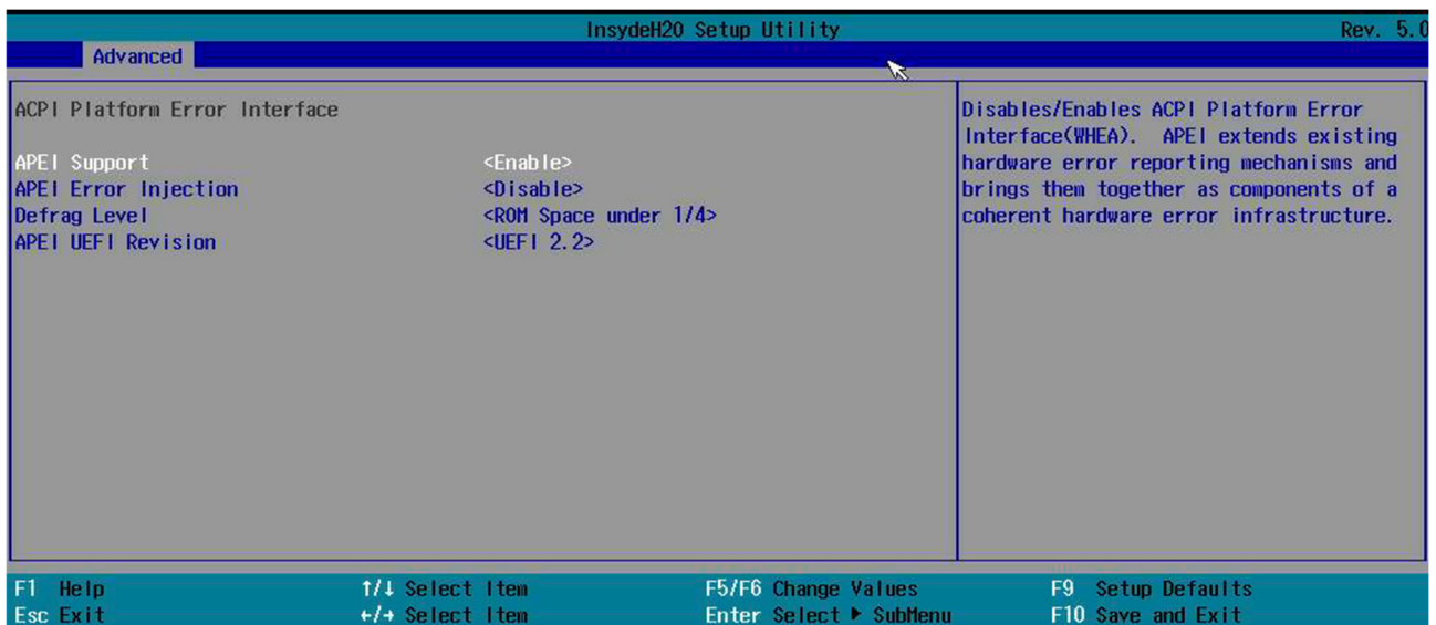
Рисунок 2.58. «APEI Configuration»
