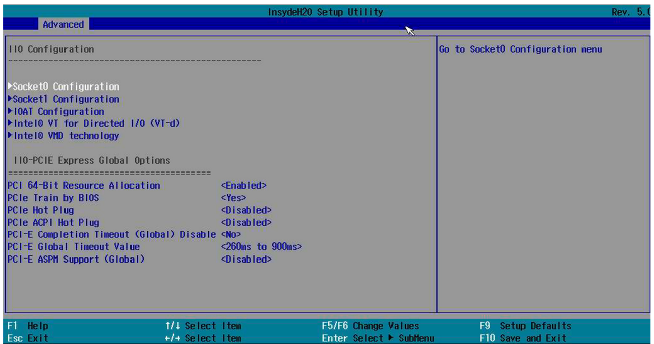
Рисунок 2.20. «I/O Configuration»
