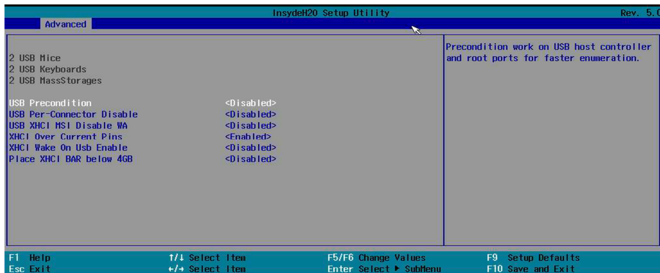
Рисунок 2.53. «USB Configuration»
