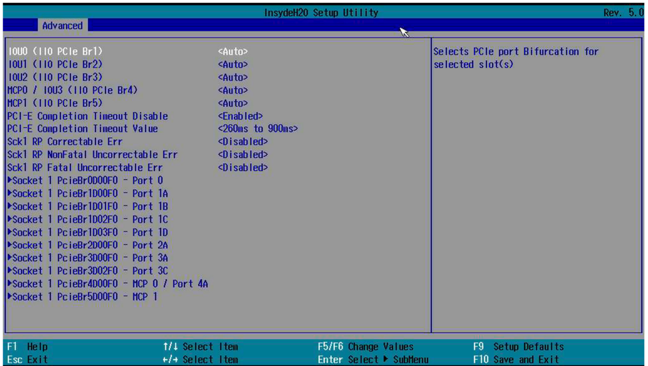
Рисунок 2.24. «Socket1 Configuration»
