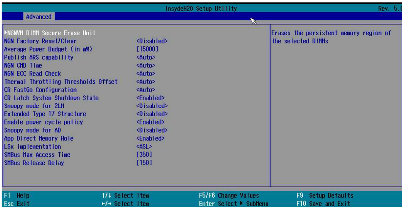
Рисунок 2.17. «NGN Configuration»
