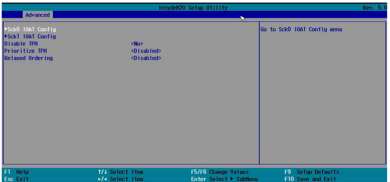
Рисунок 2.25. «IOAT Configuration»
