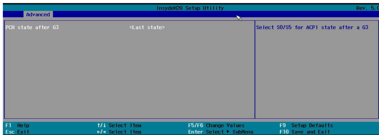
Рисунок 2.50. «PCH Devices»
