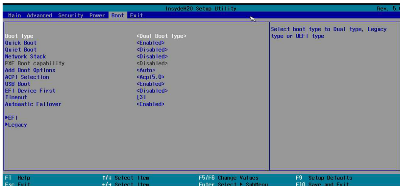
Рисунок 2.70. Вкладка «Boot»
