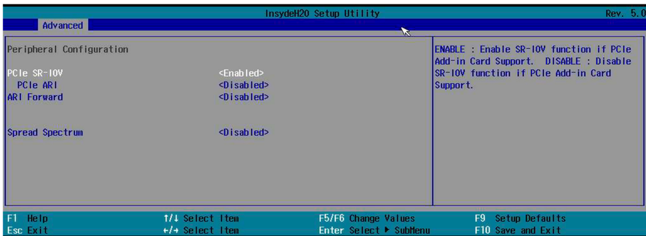
Рисунок 2.3. «Peripheral Configuration»
