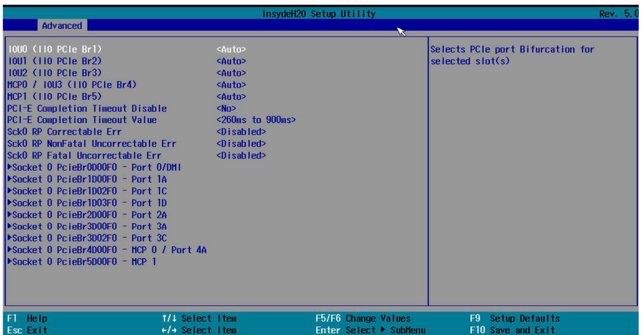
Рисунок 2.21. «Socket0 Configuration»
