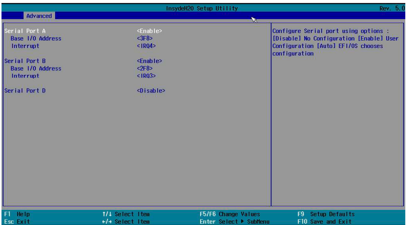
Рисунок 2.7. «SIO AST2500»
