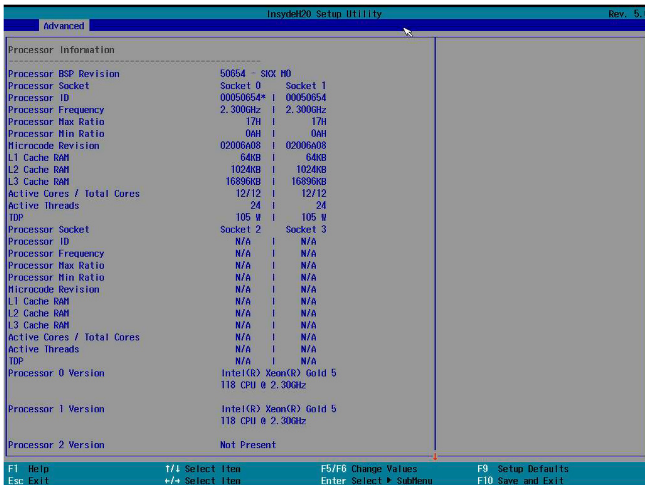
Рисунок 2.10. «Per-Socket Information»
