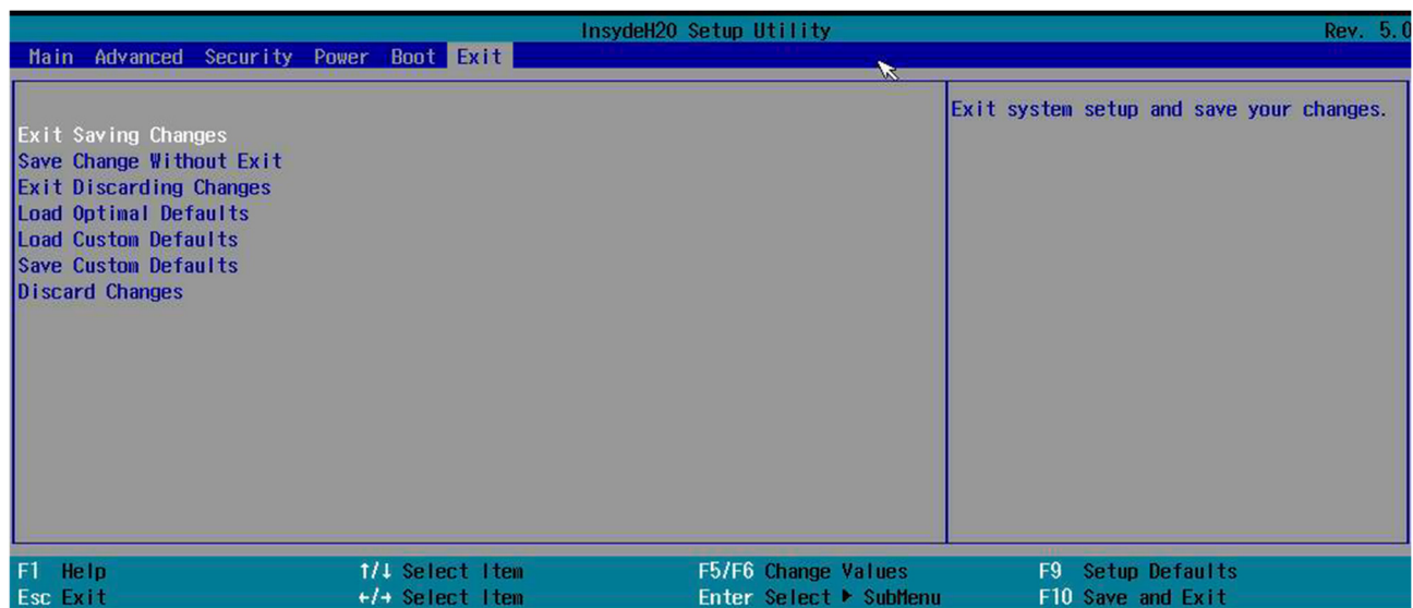
Рисунок 2.76. Вкладка «Exit»
