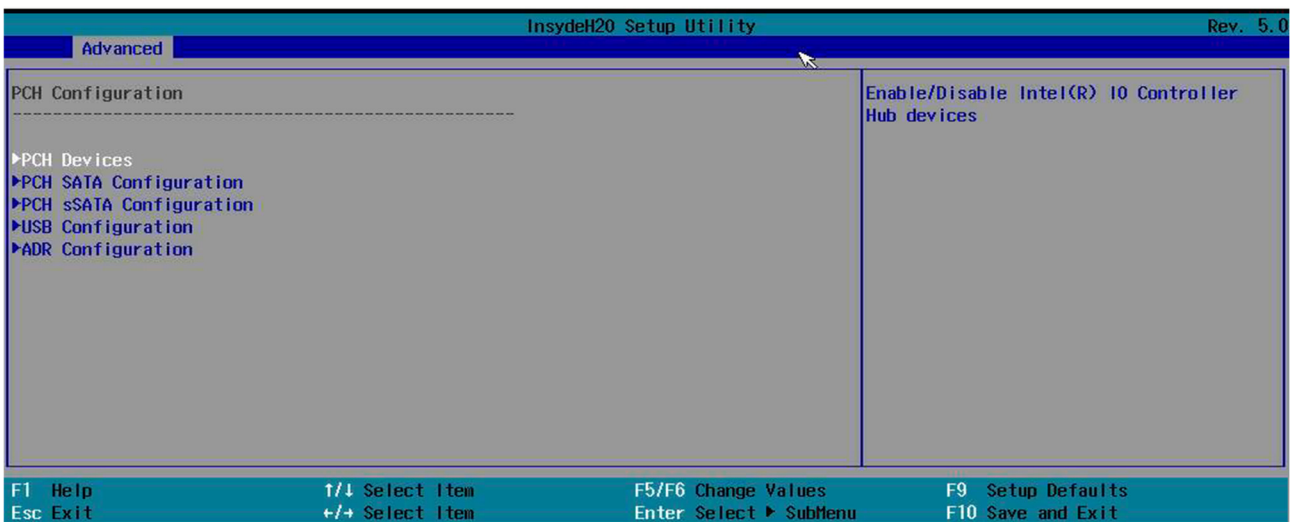
Рисунок 2.49. «Pch Configuration»
