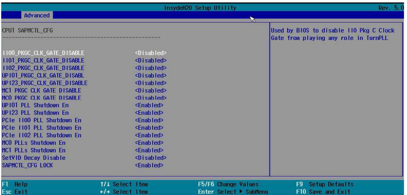
Рисунок 2.40. «CPU1 SAPMCTL_CFG»
