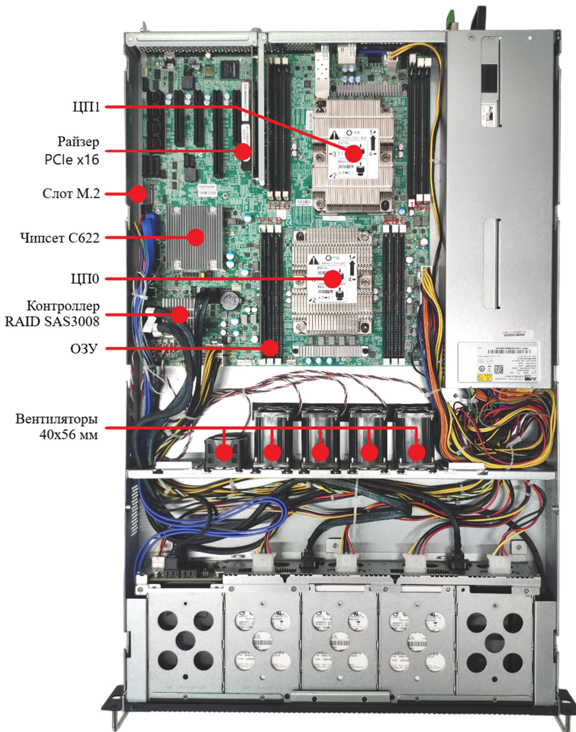
Рисунок 4. Вид сверху
