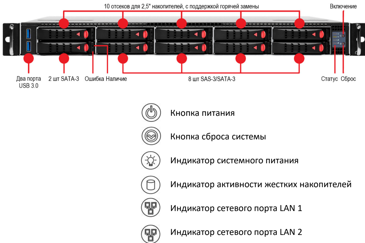
Рисунок 1. Передняя сторона
