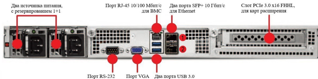
Рисунок 3. Задняя сторона
